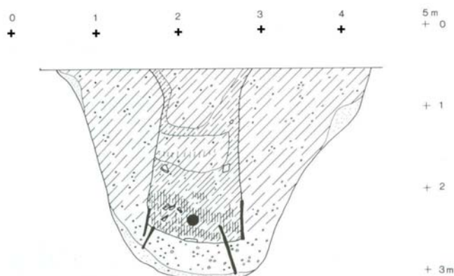
(Abb. 2) Krefeld-Hüls, Brunnen II. Profil nach Abtrag von ca. 1,5 m Boden ab Oberfläche (Kreis = Probenentnahmestelle). M 1:50
