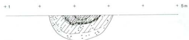
(Abb. 4) Krefeld-Hüls, Brunnen II. Planum bei 2,5 m unter 0-Linie. M 1:50
