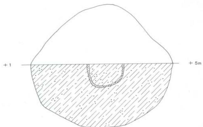
(Abb. 3) Krefeld-Hüls, Brunnen II. Planum bei 0,6 m unter 0-Linie. M 1:50
